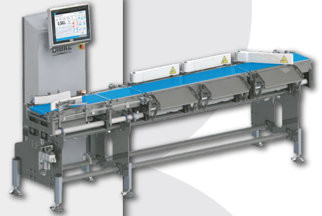
Classificadora Automática por Peso DIBAL GW-5000
