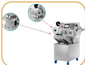
Rebobinagem do filme automática (standard) Pré-aquecimento (opcional) Câmara inferior de vácuo amovível (standard)
